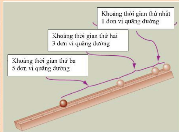
Hình 17. Mô phỏng mặt phẳng nghiêng Galilei
